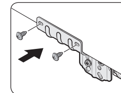
Tornillo Phillips de cabeza plana (8) - 6006-001174 (M4, L12)
