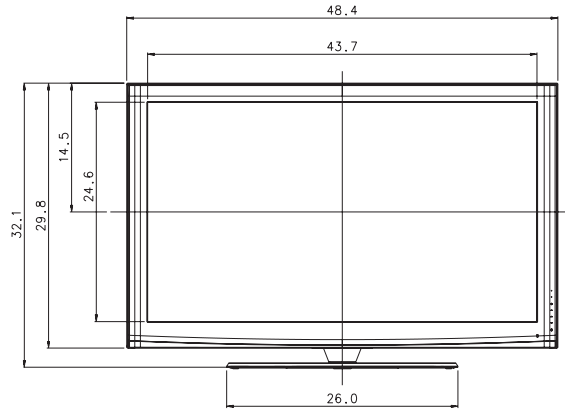
VUE AVANT
