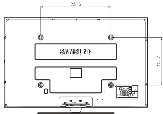
VUE ARRIÈRE
