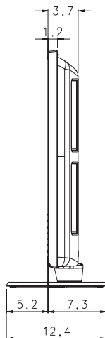
VUE LATÉRALE
