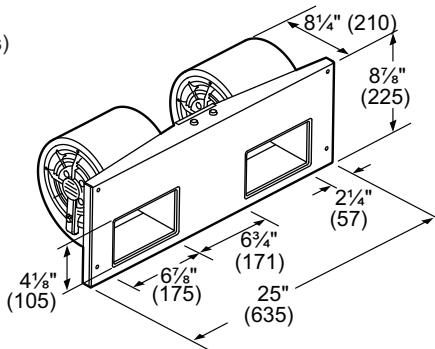
Ventilador integrado VTN1030
