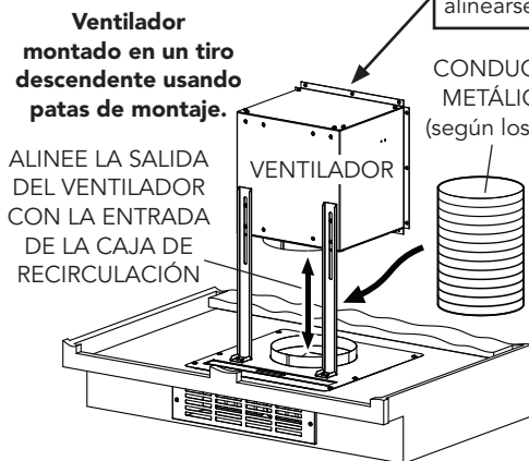
EXTRACCIÓN A TRAVÉS DEL FRENTE DEL GABINETE (ESPACIO PARA LOS PIES)
