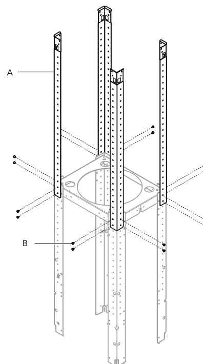
A. 4 soportes verticales superiores B. 16 tornillos de 4.2 x 8 mm
