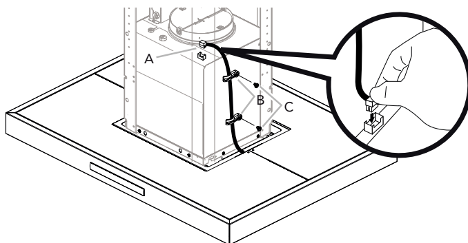
A. Conector de la campana B. Sujetacables plásticos
