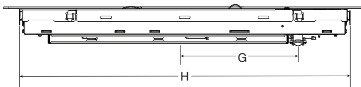
VISTA POSTERIOR
