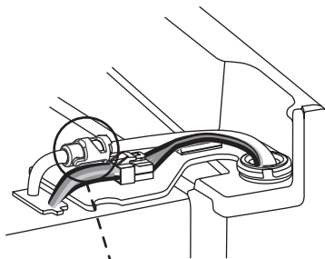
Style 2 – Raccord de tuyau du distributeur d'eau
