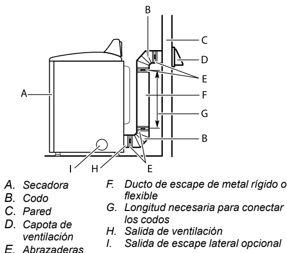
Instalación por la parte superior (también está disponible con un codo de desviación)
