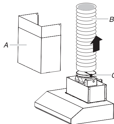
A. Cubiertas de ventilación B. Sistema de ventilación C. Pieza de transición del ducto
