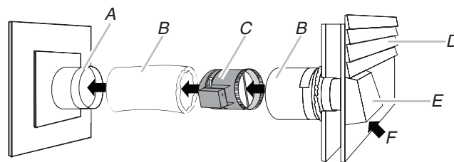
A. Bouche murale B. Conduits C. Clapet motorisé de 6" (15,2 cm)
