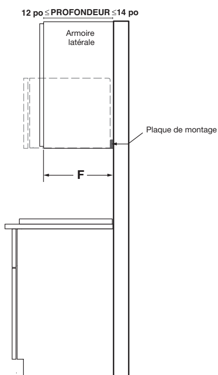
VUE LATÉRALE
