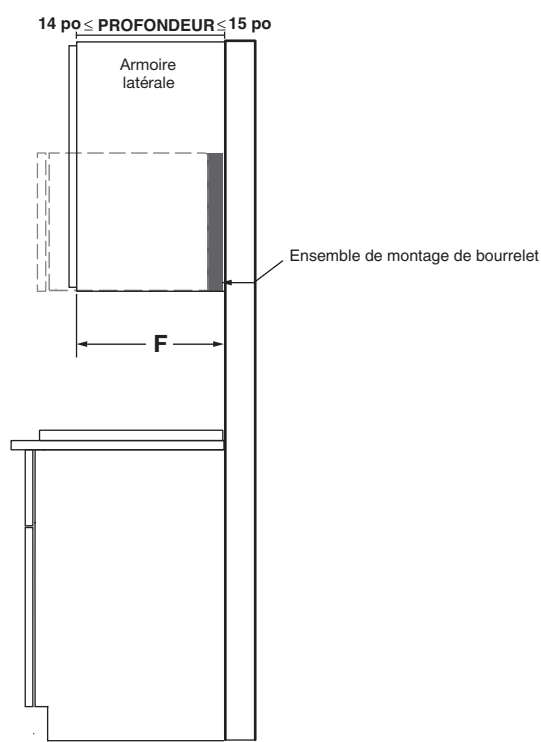
VUE LATÉRALE
