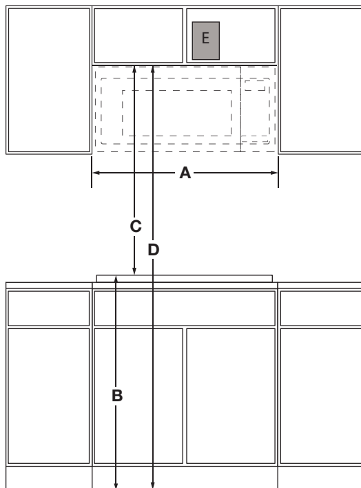
VUE AVANT
