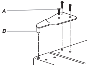
A. Vis de charnière à tête hexagonale de \frac{5}{16} " B. Charnière supérieure
