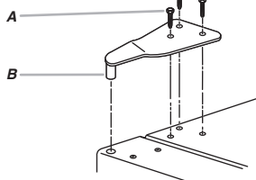
A. 1/16" Hex-Head Hinge Screws B. Top Hinge
